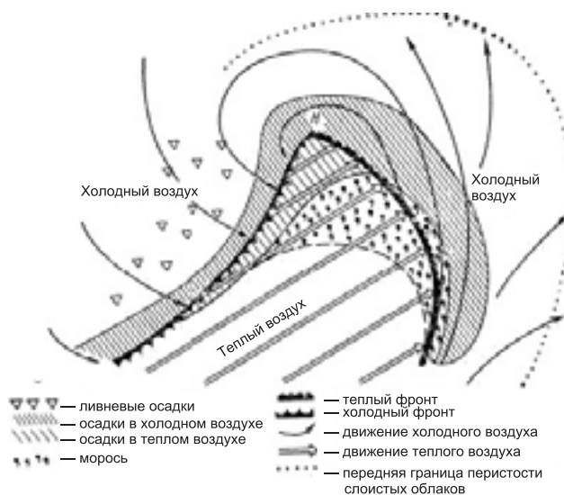
Рис. 2. Схема строения типичного циклона
